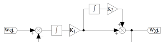
Rys.3. Proponowana struktura obserwatora ATO dla fizycznego estymatora położenia kątoowego
