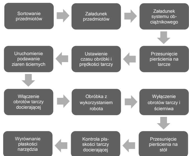
Rys. 5. Zasada działa systemu docierania z wykorzystaniem robota
