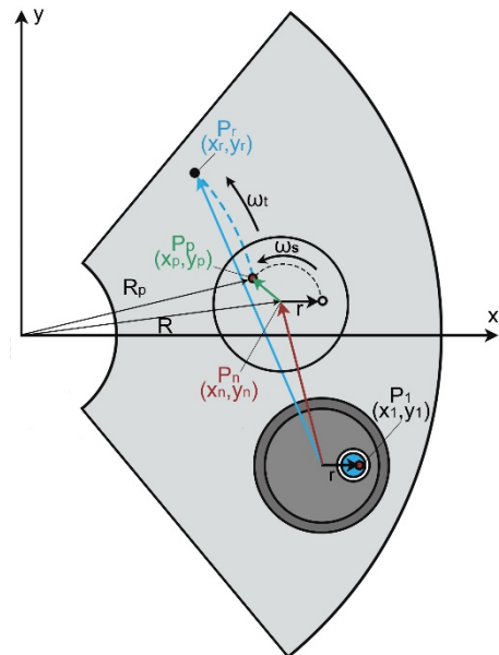
Rys. 10. Schemat interpolacji kołowej
