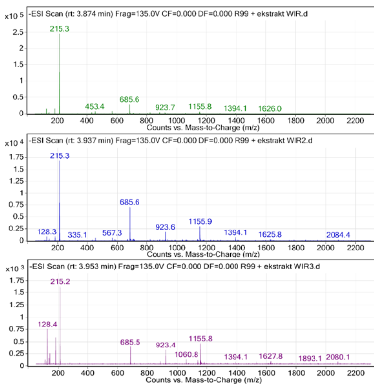
Rys.81. Widma masowe związku K-Lip-1, który został poddany działaniu ekstraktu bezkomórkowego (czas trwania hydrolizy: 0, 40 i 120 minut).
