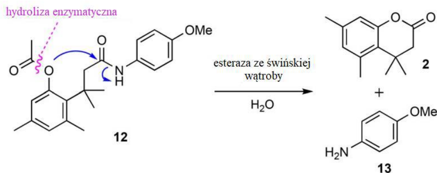
Rys.4. Mechanizm działania hydrolizy enzymatycznej TML pod wpływem esterazy [18]. Wskutek działania esterazy następuje reakcja laktonizacji estru acetylowego TML (12), co wiąże się z uwolnieniem p-metoksyaniliny (13) z układu.
