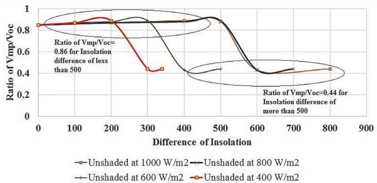
Rys. 9. Przesunięcie GMPP przy różnym nasłonecznieniu [tłum. Ratio of V_{mp}/V_{oc} – Stosunek V_{mp}/V_{oc} , Ratio of V_{mp}/V_{oc} = 0.86 for Insolation difference of less than 500, Ratio of V_{mp}/V_{oc} = 0.44 for Insolation difference of more than 500 – stosunek V_{mp}/V_{oc} = 0,44 przy różnicy nasłonecznienia większej niż 500, Difference of Insolation – Różnica nasłonecznienia, Unshaded at 1000 W/m^2 – niezacieniony przy 1000 W/m^2 , Unshaded at 600 W/m^2 – niezacieniony przy 600 W/m^2 , Unshaded at 800 W/m^2 – niezacieniony przy 800 W/m^2 , Unshaded at 400 W/m^2 – niezacieniony przy 400 W/m^2 ]
