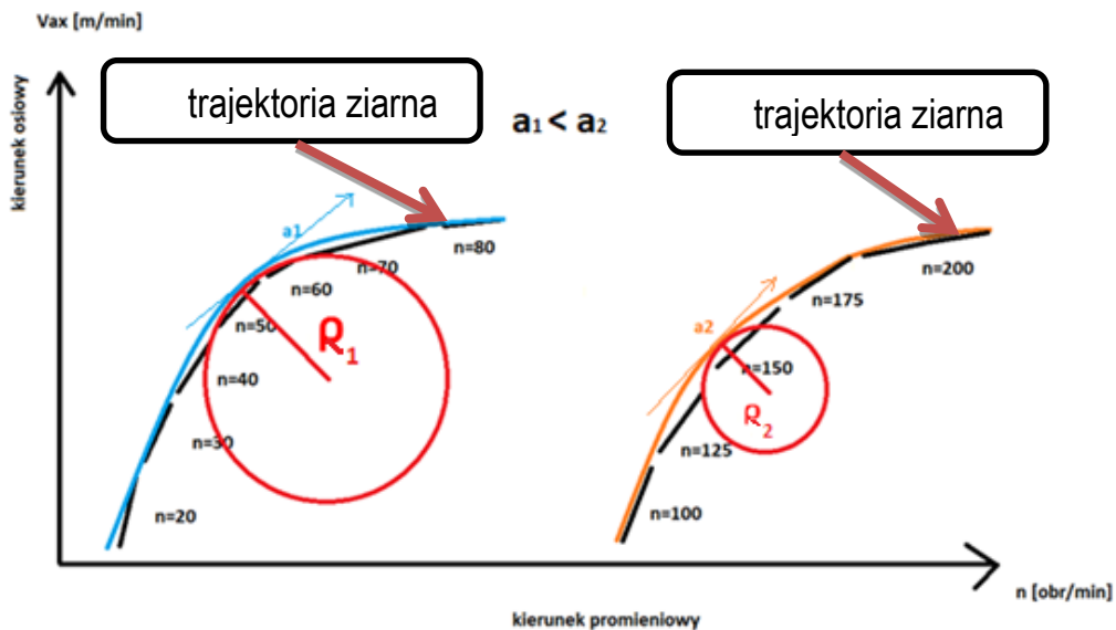
Rys. 228. Trajektorja ziarna z większym promieniem R_1 krzywej K dla zmiany prędkości obrotowej w zakresie n = 20 \div 80 obr/min, trajektorja ziarna z mniejszym promieniem R_2 krzywej K dla zmiany prędkości obrotowej w zakresie n = 100 \div 200 obr/min
