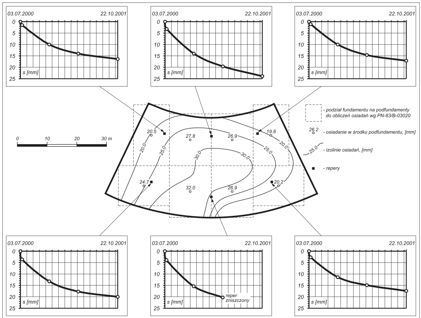
Rys. 9 Porównanie osiadań obliczonych metodą odkształceń jednoosiowych z pomiarami geodezyjnymi (budynek PPPL)
