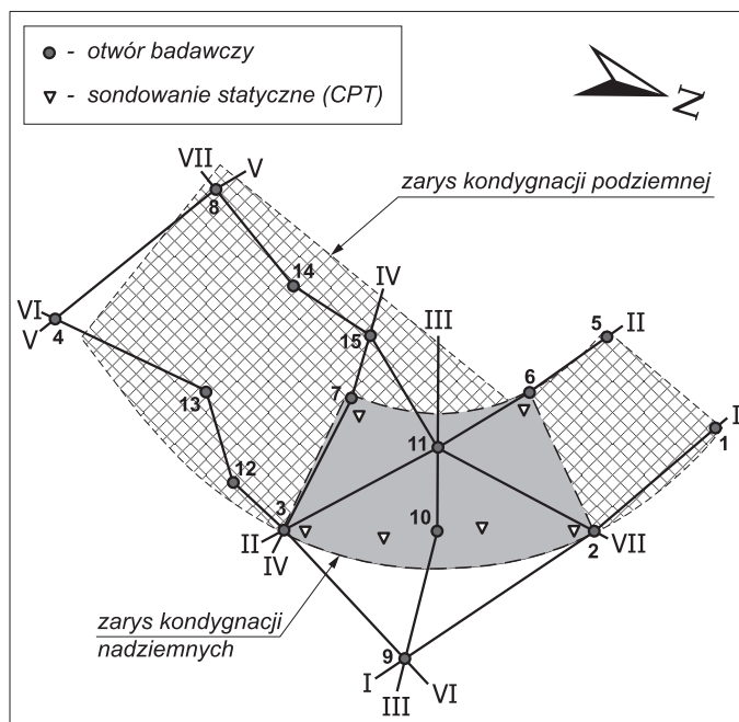
Rys. 5 Usytuowanie wiercni badawczych i sondowań statycznych pod budynek PPPL
