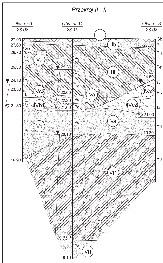
Rys. 6 Fragment przekroju II-II (budynek PPPL)
