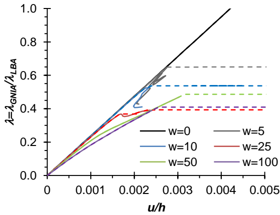
Rys. 6.68. Silos A: zależność mnożnika obciążenia \lambda_{GNIA}/\lambda_{LBA} od względnego skrócenia silosu u/h dla różnych amplitud imperfekcji w [mm] (1 postać wyboeczeniowa) na podstawie nieliniowej analizy statycznej (—) i dynamicznej (- - -)
