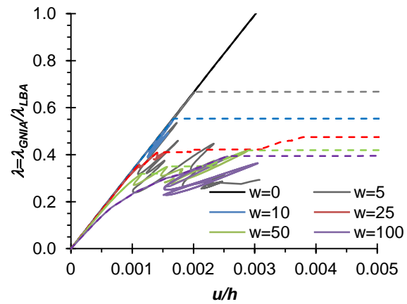
Rys. 6.68. Silos A: zależność mnożnika obciążenia \lambda_{GNIA}/\lambda_{LBA} od względnego skrócenia silosu u/h dla różnych amplitud imperfekcji w [mm] (1 postać wyboeczeniowa) na podstawie nieliniowej analizy statycznej (—) i dynamicznej (- - -)
