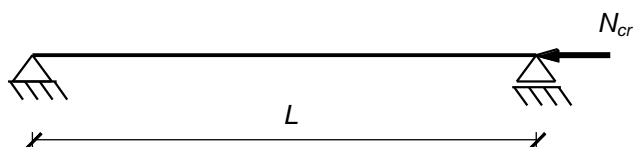
Rys. 6.15. Schemat statyczny ściskanego pręta
