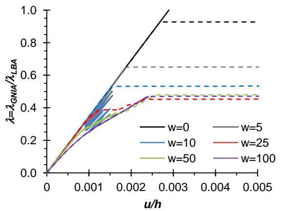
Rys. 6.69. Silos B: zależność mnożnika obciążenia \lambda_{GNIA}/\lambda_{LBA} od względnego skrócenia silosu u/h dla różnych amplitud imperfekcji w [mm] (1 postać wyboeczeniowa) na podstawie nieliniowej analizy statycznej (—) i dynamicznej (- - -)
