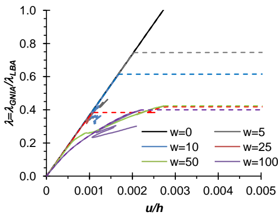
Rys. 6.69. Silos B: zależność mnożnika obciążenia \lambda_{GNIA}/\lambda_{LBA} od względnego skrócenia silosu u/h dla różnych amplitud imperfekcji w [mm] (1 postać wyboeczeniowa) na podstawie nieliniowej analizy statycznej (—) i dynamicznej (- - -)
