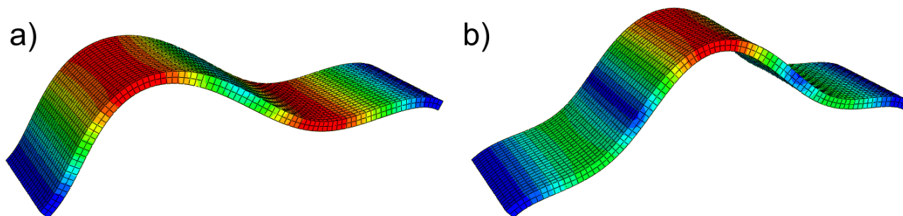
Rys. 92 Pierwsza (a) i druga (b) postać drgań własnych wg opracowania autora.
