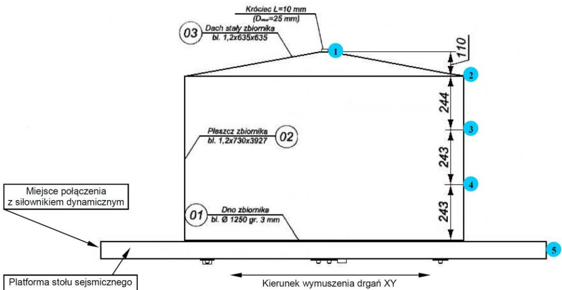
Rys. 3.9. Rozmieszczenie punktów pomiarowych przyspieszeń w badaniach modelu zbiornika o średnicy D=1,25\text{ m}
