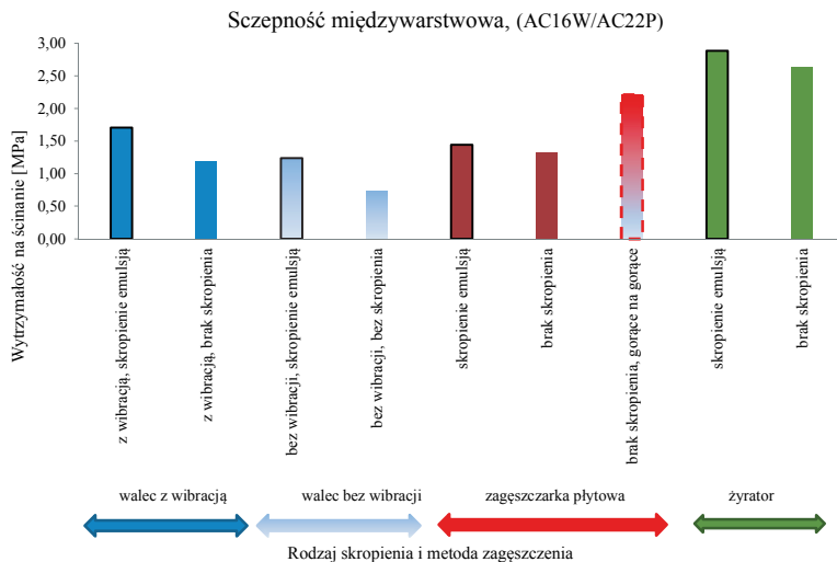
Rys. 3. Wyttrzymałość na ścinanie próbek przygotowanych w laboratorium różną metodą zagęszczenia i z różną warstwą szepną
