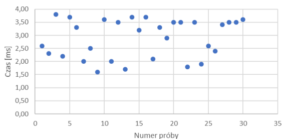
Rys. 6. Czasy round-trip dla przełącznika CB1
