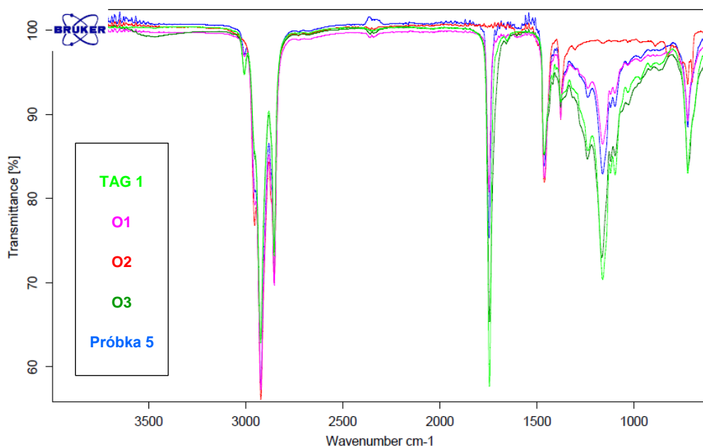
Rysunek A4-8. Nałożone widma FT-MIR dla: TAG1– olej roślinny, rzepakowy, jadalny; O1 - olej do smarowania łańcuchów pilarek, mieszanka olejów pochodzenia naftowego oraz roślinnego; O2- olej maszynowy, mineralny; O3- w pełni biodegradowalny olej do smarowania łańcuchów pilarek; próbka 5
