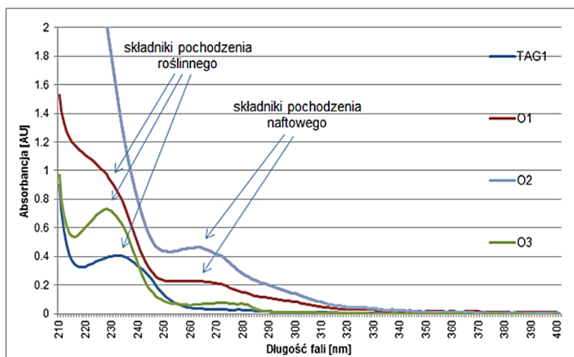
Rysunek A4-2. Nałożone widma UV 4 próbek olejów odniesienia o stężeniu 0,25 mg oleju /ml n-heksanu dla zakresu długości fal od 210-400 nm (TAG1 – olej roślinny, rzepakowy, jadalny, O1-olej smarowy produkowany na bazie mieszaniny oleju roślinnego oraz naftowego, O2- olej maszynowy, mineralny, O3- olej smarowy produkowany na bazie roślinnej z dodatkami uszlachetniającymi)
