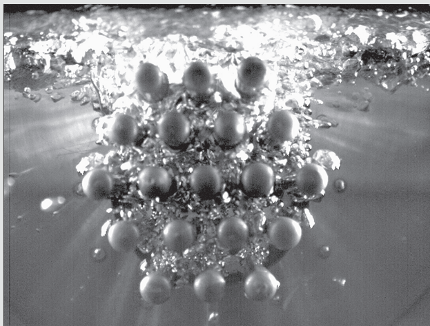
Rys. 10. Wizualizacja intensyfikującego oddziaływania pęcherzyków pary dla wrzenia wody na pęku rur o s/d = 1,7 , przy ciśnieniu atmosferycznym ( p = 100,5 \text{ kPa} ) i gęstości strumienia ciepła q = 30,25 \text{ kW/m}^2
