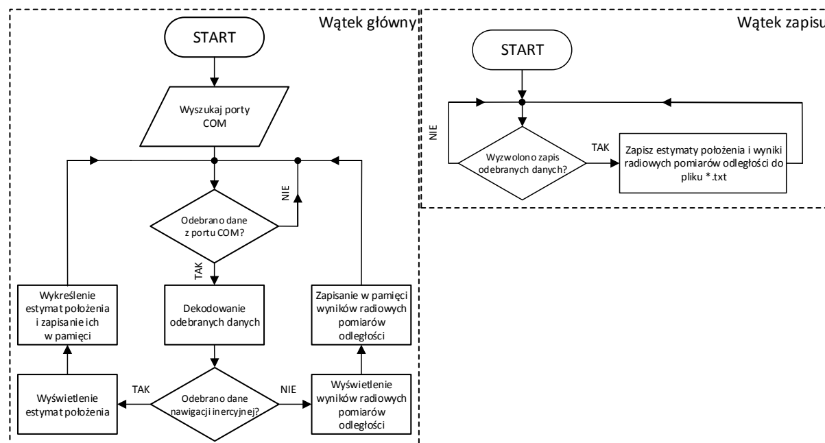
Rys. 5.7. Algorytm przetwarzania danych w aplikacji serwer_SRP .
