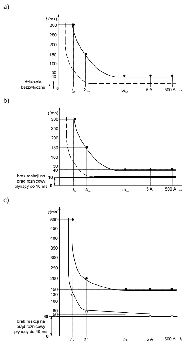
Rys.3. Charakterystyki czasowo-prądowe wyłączników różnicowoprądowych: a) bezzwłoczny, b) krótkozwłoczny (brak reakcji na prąd różnicowy płynący do 10 ms), c) selektywny (brak reakcji na prąd różnicowy płynący do 40 ms)
