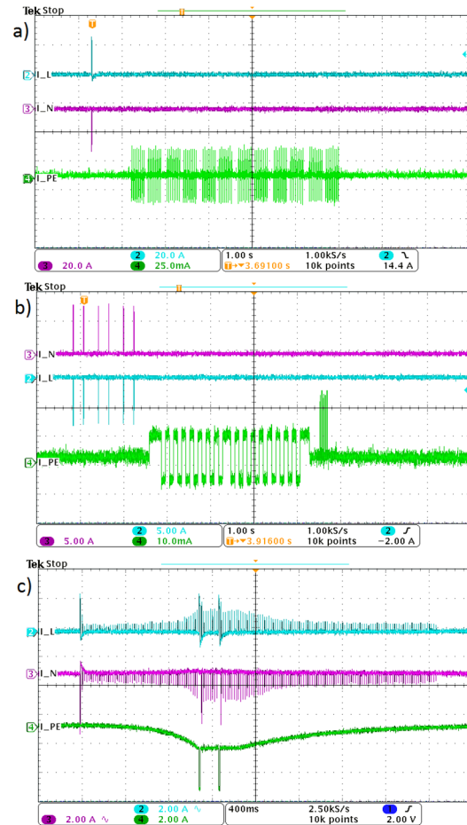
Rys. 4.2 Przebiegi prądów w przewodach L, N i PE podczas pomiaru z aktywną funkcją ATT/RCD, a) Sonel MPI-520 (skala: I_L, I_N - 20\text{A/dz.}, I_{PE} - 25\text{mA/dz.} ), b) Kyoritsu KEW 4140 (skala I_L, I_N - 5\text{A/dz.}, I_{PE} - 10\text{mA/dz.} ), c) Kyoritsu 4120A (skala 2A/dz.)
