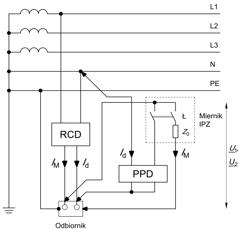
Rys. 5.4 Schemat układu pomiaru impedancji pętli bez wyzwalania RCD z przetwornikiem prądu dopełniającego PPD połączony równolegle do zacisków badanego odbiornika [85]
