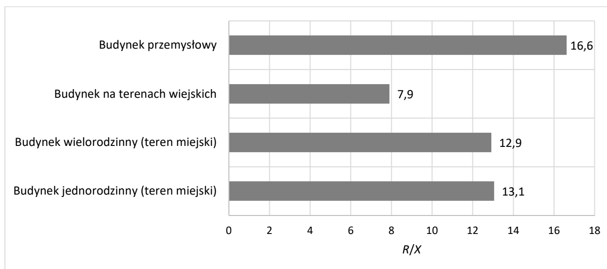
Rys. 3.7 Wykres wartości stosunku R/X dla różnych typów symulowanych sieci
