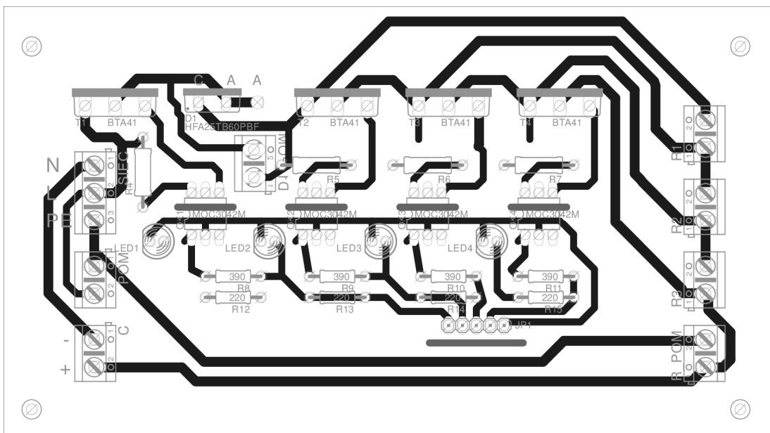
Rys. 7.2 Schemat płytki drukowanej nowej wersji miernika rezystancji pętli zwarciowej
