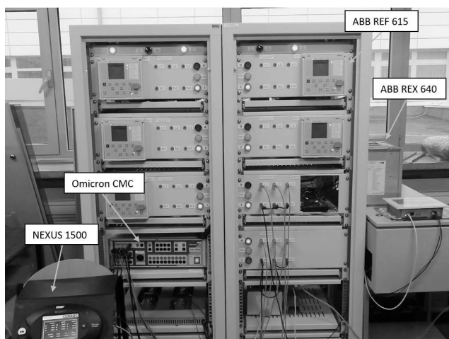
Rys. 4. Stanowisko badawcze
