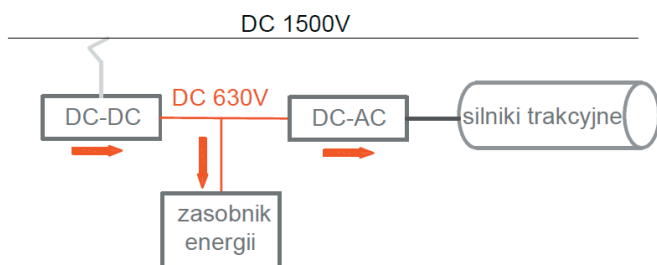
Rys. 2. Przykładowy schemat zasilania i ładowania zasobników w pojeździe
