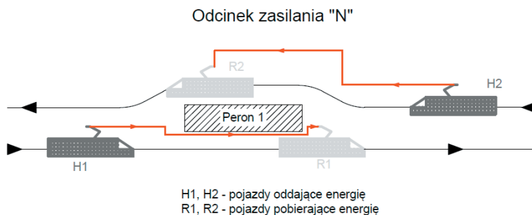
Rys. 3. Uproszczony schemat rekuperacji energii w systemie pojazd - pojazd w rejonie posterunku ruchu Źródło: opracowanie własne
