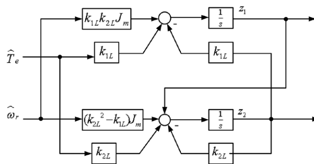
Rys. 3. Struktura obserwatora momentu obciążenia.
