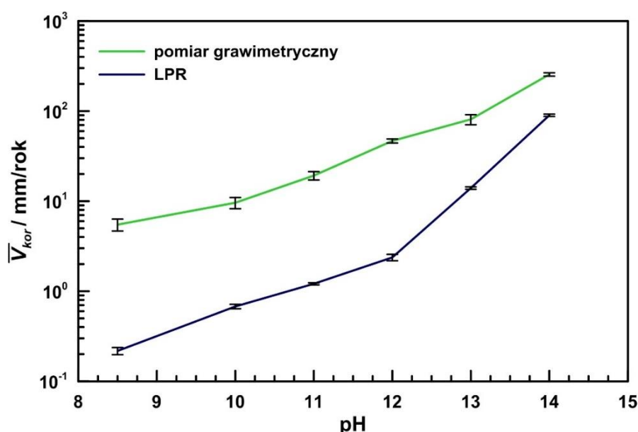
Rys. 60. Zmiany szybkości korozji w funkcji pH elektrolitu \overline{V}_{kor} = f(\text{pH}) dla stopu aluminium AA1050 wyznaczone na podstawie pomiarów grawimetrycznych (wartość średnia z 5 pomiarów) i LPR (wartość średnia z 30 cykli pomiarowych).
