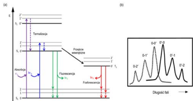
Rys. 3. Schemat poziomów energetycznych w materiałach luminesujących (a) oraz widmo luminescencji będące wynikiem przejść singletowych i oscylacyjnych (b). Z lewej strony pokazany jest schemat Jabłońskiego, z prawej widmo absorpcyjne (linia przerywana) i widmo emisyjne (linia ciągła) wynikające z schematu Jabłońskiego, z włączeniem struktury oscylacyjnej.
