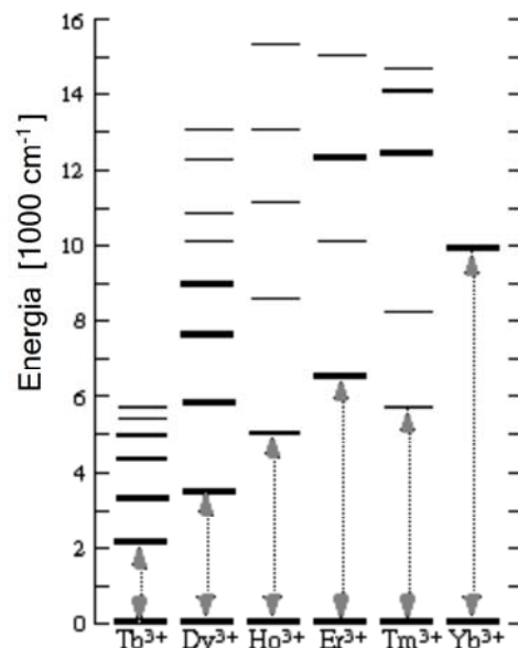
Rys. 9. Jony ziem rzadkich wykorzystywane jako domieszki w szklach do chłodzenia w wyniku luminescencji antystokesowskiej [10]
