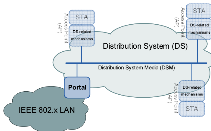
Fig. 6 IEEE 802.11 Portal
