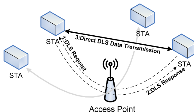
Fig. 18 Direct Link Protocol.
