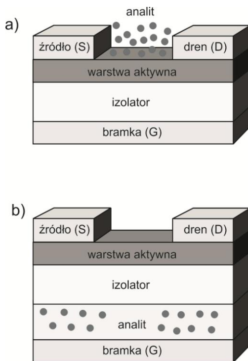
Rysunek 8. Schematy detektorów OFET w których: a) analit pozostaje w bezpośrednim kontakcie z aktywną warstwą tranzystora; b) działaniu badanego analitu poddawana jest elektroda bramkująca [opracowanie własne na podstawie [4]]
