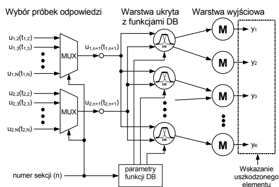
Rys. 6. Architektura klasyfikatora DB do lokalizacji uszkodzeń w wielosekcyjnym torze analogowym Fig. 6. Architecture of the DB classifier for localization of faults in a multisecton analog path
