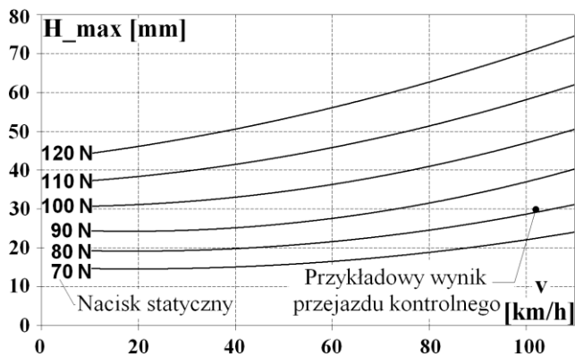
Rys. 17. Charakterystyki uniesienia przewodu jezdny w zależności od siły statycznej odbieraka i prędkości pojazdu
