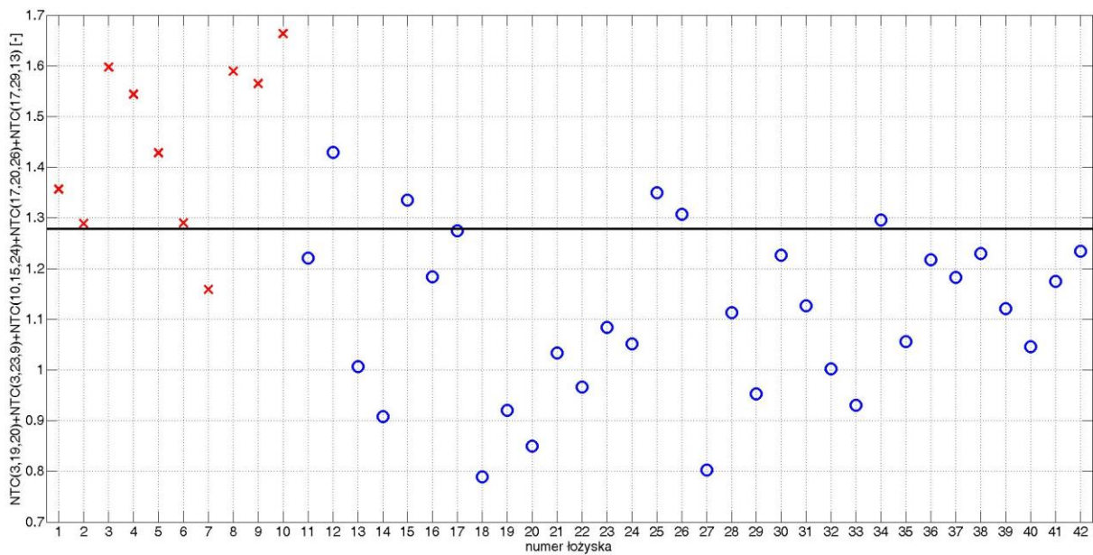
Rys. A. 28. Wartość wskaźnika diagnostycznego dla poszczególnych łożysk dla zestawu 4 przy obciążeniu 0,6 kW
