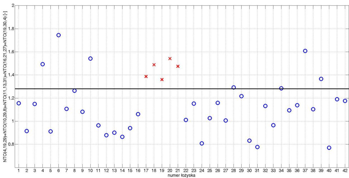
Rys. C. 6. Wartość wskaźnika diagnostycznego dla poszczególnych łożysk dla zestawu 2 przy obciążeniu 1,0 kW
