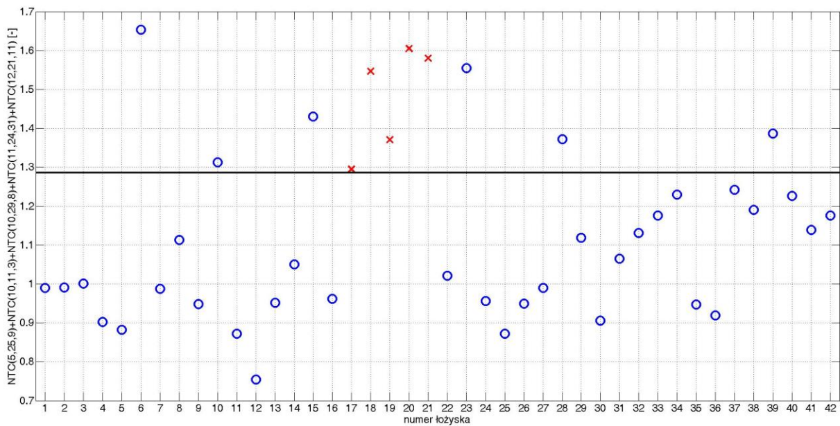
Rys. C. 8. Wartość wskaźnika diagnostycznego dla poszczególnych łożysk dla zestawu 4 przy obciążeniu 1,0 kW
