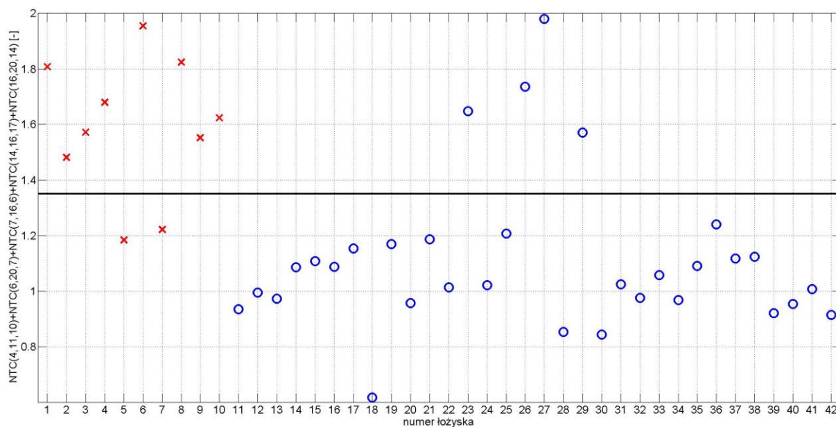
Rys. A. 2. Wartość wskaźnika diagnostycznego dla poszczególnych łożysk dla zestawu 3 przy obciążeniu 1,1 kW
