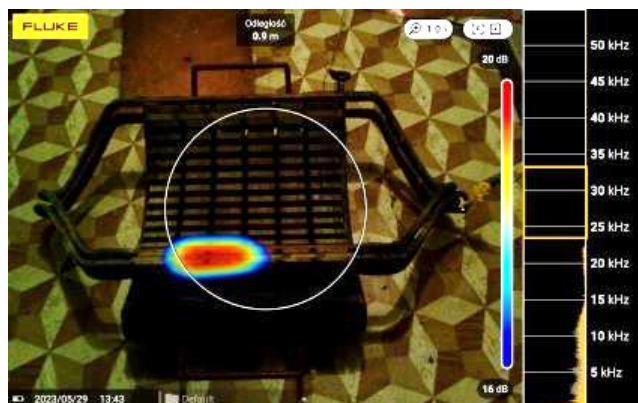
Rys. 6. Lokalizacja WNZ w cewce z 1973 roku przy napięciu przemiennym 3,5 kV (znamionowe napięcie fazowe U_{IN} = 3,46 kV)
