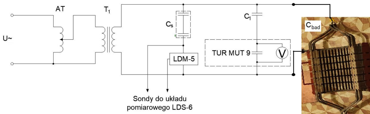
Rys. 5. Schemat układu pomiarowego, U\sim - napięcie wejściowe, AT - autotransformator, T_1 - transformator, C_1 - kondensator WN dzielnika 60 pF, C_s - kondensator sprzęgający 2 \times 1000 pF, TUR MUT 9 - układ pomiarowy, C_{bad} - pojemność obiektu badanego
