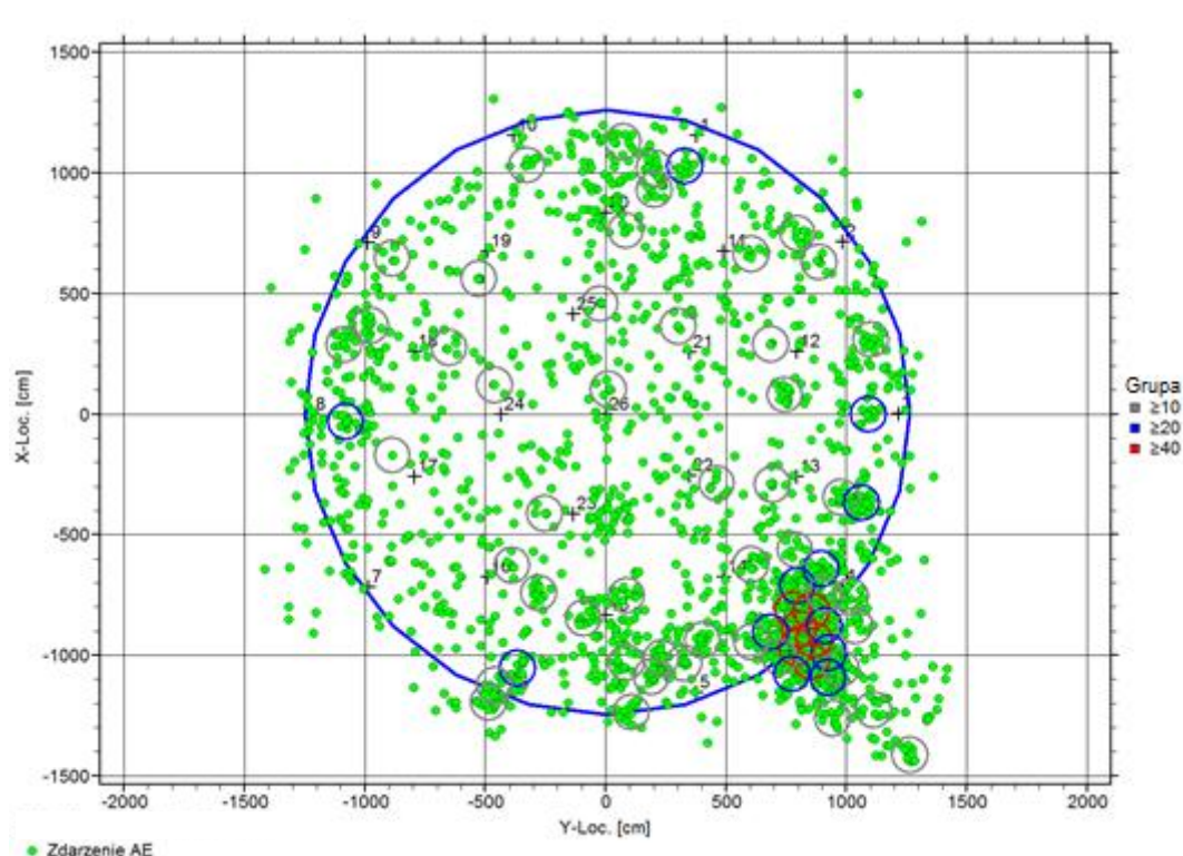
Rys. 5.7. Lokalizacja źródeł AE na dnie zbiornika magazynowego V = 9600 \text{ m}^3
