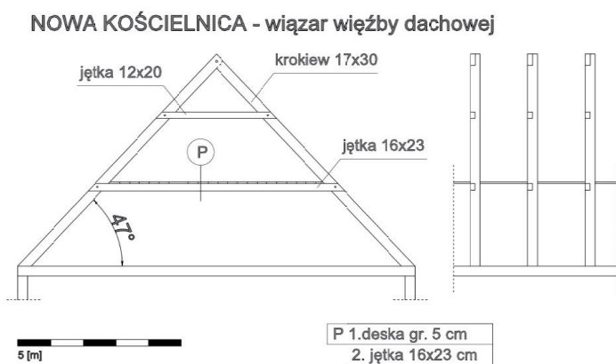
Rys. 4. Uproszczony schemat więźby dachowej domu podcieniowego Nowej Kościelnicy. (opracowanie autora)
