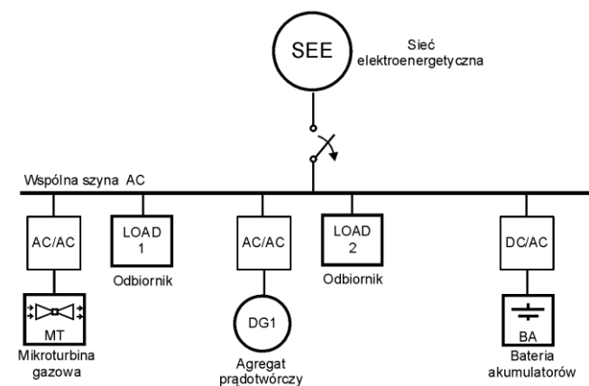
Rys. 5 Mikro sieć z baterią akumulatorów i możliwością współpracy z siecią elektroenergetyczną
