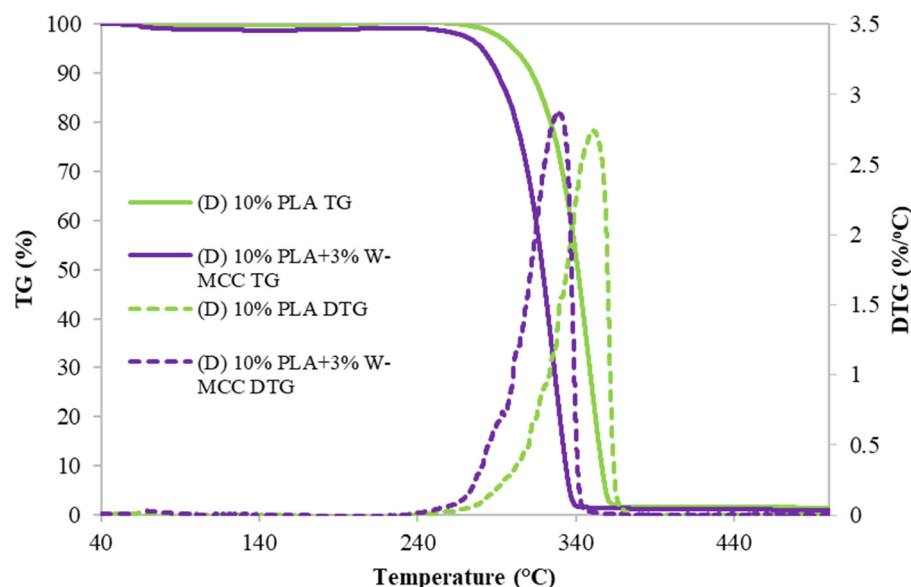
Figure 6. TG and DTG profiles of (D) 10% PLA and (D) 10% PLA+3% W-MCC.
