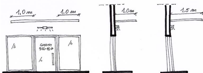
Rysunek 5. Wymagania dla zadaszenia, 1,0 m dla budynków niskich i 1,5 m dla budynków wysokich (Figure 5. Requirements for a of small roof—1.0 m for low buildings and 1.5 m for high buildings)
