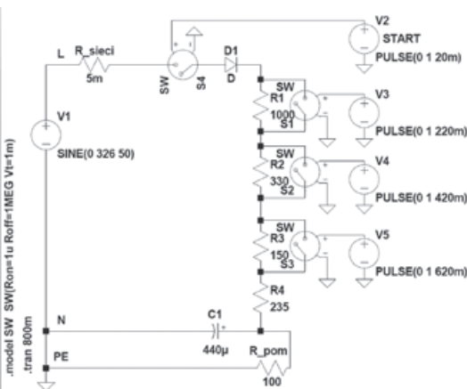
Rys. 10. Schemat ideowo-symulacyjny proponowanego układu pomiaru impedancji (rezystancji) pętli zwarciowej (a) oraz uzyskany z symulacji przebieg prądu pomiarowego (b)
