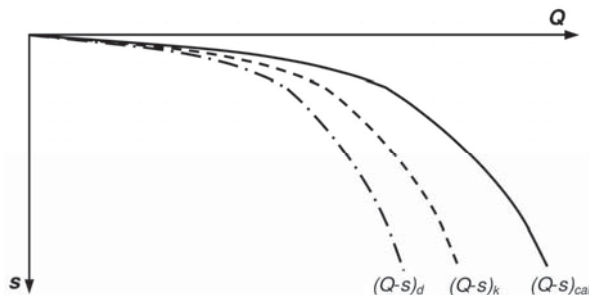
Rys. 9. Charakterystyki Q-s pała: obliczona, charakterystyczna i projektowa Fig. 9. Load-settlement curves of pile: calculated, characteristic and design
