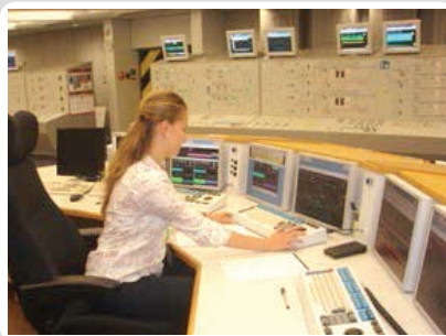
Fot. 3. Symulator nastawni elektrowni jądrowej
