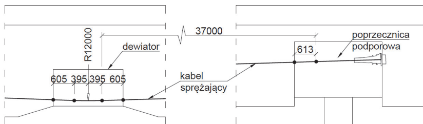
Rys. 2. Schemat przebiegu i warunki brzegowe dla kabla przy przejściu przez dewiator i w zakotwieniu
