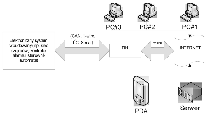
Rys. 1. Schemat blokowy aplikacji na platformie TINI
