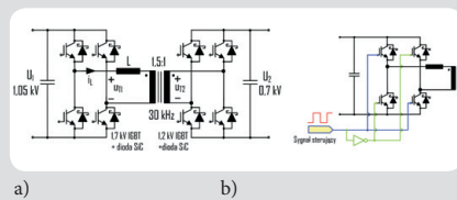
Rys. 4. Sterowana przetwornica izolowana DC-DC z tranzystorami IGBT i diodami zwrotnymi z węgla krzemu (SiC) (a); sposób rozdzielania sygnału sterującego tranzystorami mostka (b)
