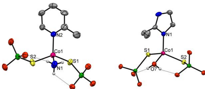
Rys. 3.20. Struktura molekularna związków o wzorze [\text{Co}\{\text{SSi}(\text{O}t\text{Bu})_3\}_2(\text{NH}_3)(2\text{-Mepy})] (lewa strona) oraz [\text{Co}\{\text{SSi}(\text{O}t\text{Bu})_3\}_2(2\text{-Etim})(\text{H}_2\text{O})] (prawa strona). Wiązania wodorowe oznaczono cienką szarą linią. Dla czytelności rysunku pomięto wybrane atomy wodoru oraz grupy tert -butylowe. Elipsoidy drgań termicznych 30% [97, 99].
