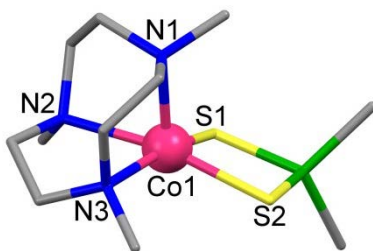
Rys. 3.15. Struktura molekularna związku o wzorze [Co(Me 3 TACN)(S 2 SiMe 2 )]. Dla czytelności rysunku pominięto atomy wodoru [65].
