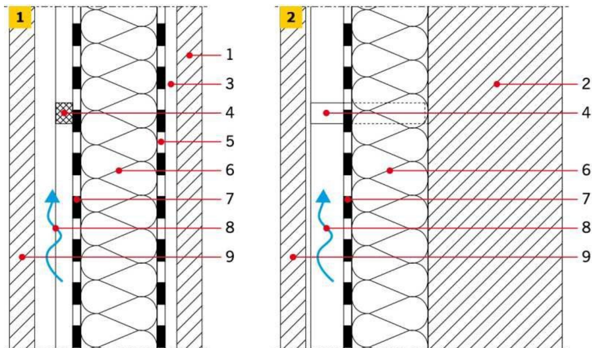
RYS. 1-2. Przykłady zastosowania materiałów okładzinowych w przegrodzie budowlanej typu ściana osłonowa (1) i typu okładzina ścienna (2): 1 - okładzina wewnętrzna, 2 - ściana konstrukcyjna, 3 - konstrukcja nośna przegrody, 4 - podkonstrukcja nośna okładziny, 5 - warstwa izolacji paroszczelnej, 6 - warstwa izolacji termicznej, 7 - warstwa izolacji wiatroszczelnej, 8 - wentylowana pustka powietrzna, 9 - materiał okładziny zewnętrznej (elewacyjnej); rys. archiwum autora
