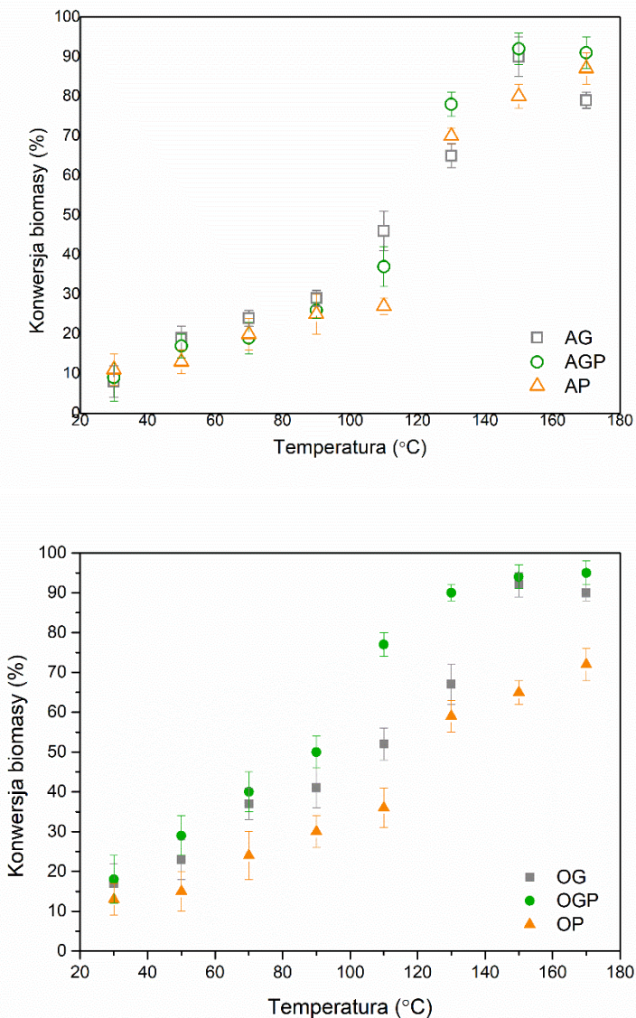
Rysunek 19. Zależność konwersji biomasy od temperatury w trakcie procesu upłynniania.
