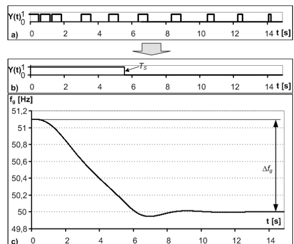
Rys. 1. Istota metody MASD [6]: a) impulsy sterujące – typowy SA, b) impuls sterujący wg MASD, c) zmiana częstotliwości zadanej łączonego obiektu Fig. 1. The essence of the MASD method: a) control signals – typical SA, b) control signals according to MASD, c) change of the input frequency of a connected object
