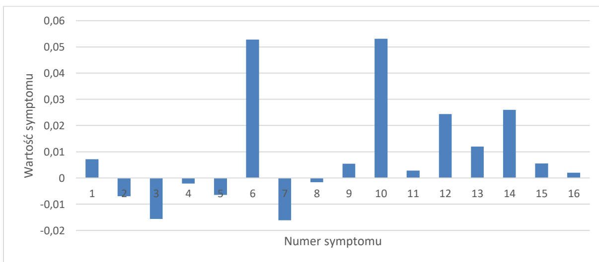
Rys. 60 Syndrom dla poszukiwania poczwórnej degradacji (11% krawędzi spływowych profili 6 GS SP, 61% luzu w uszczelnieniach 4 GS SP, 31% luzu w uszczelnieniach 2 GS WP i 7 % luzu w uszczelnieniu zewnętrznym kadłuba SP, 11% zmianę luzu w uszczelnieniu skrzynki dyszowej zaworu regulacyjnego SP, 22% luzu w uszczelnieniach 6 GS SP).
