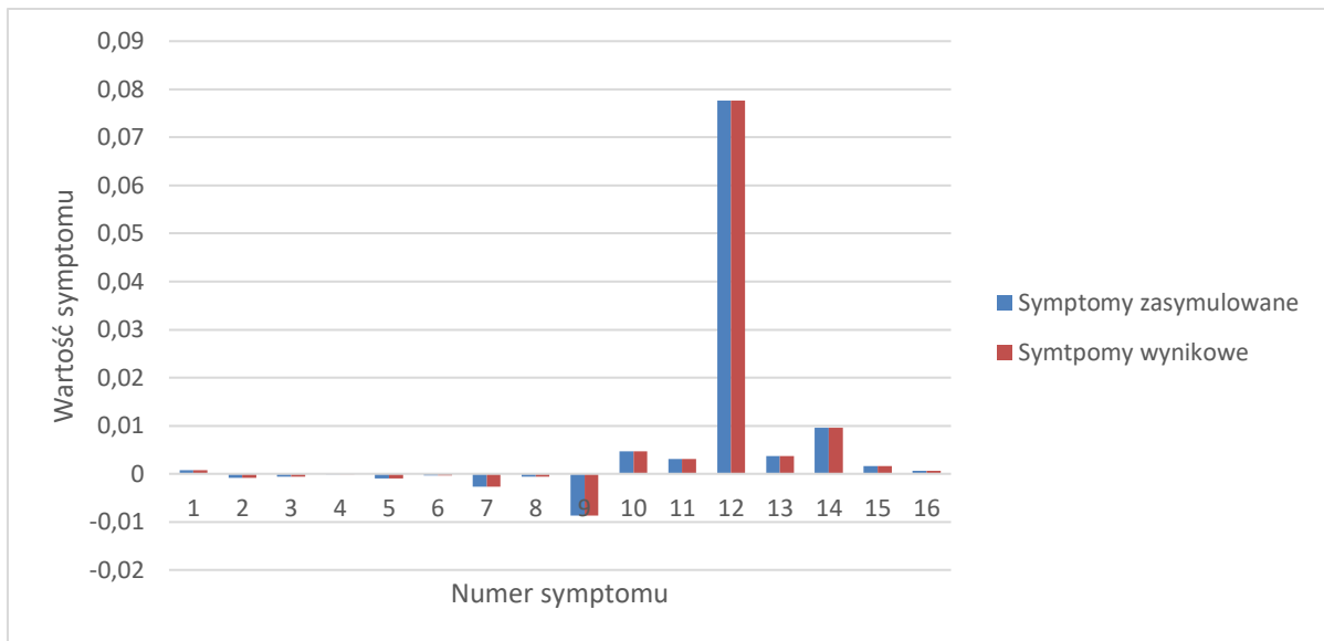
Rys. 25 Porównanie otrzymanych charakterystyk degradacji oraz poszukiwania jej dla luzu w uszczelnieniach 5 GS SP.
