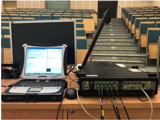
Rysunek 6-17 Sprzęt pomiarowy wykorzystany podczas badań: system PULSE (po lewej), analizator NTI AL1 (po prawej)
