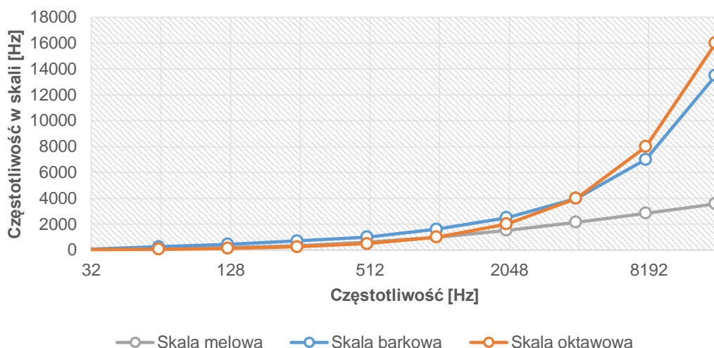
Rysunek 5-24 Zestawienie skal częstotliwościowych
