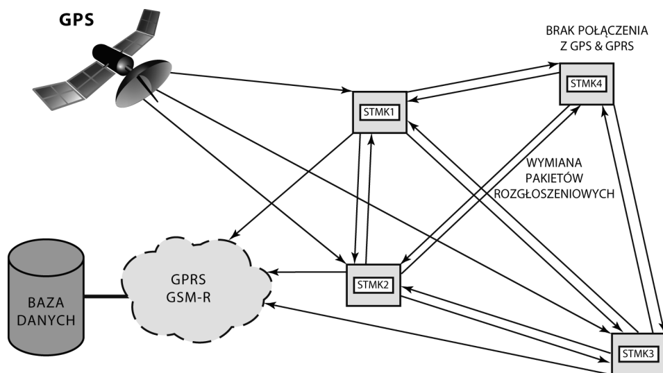
Rys. 5. Przykładowa konfiguracja sieci monitorującej przed procesem samoorganizacji
