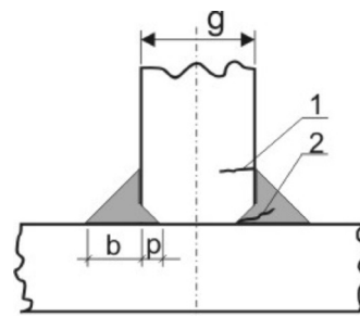
Rys. 7. Charakterystyka geometryczna złącza krzyżowego Fig. 7. Geometrical characteristics of cruciform joints
