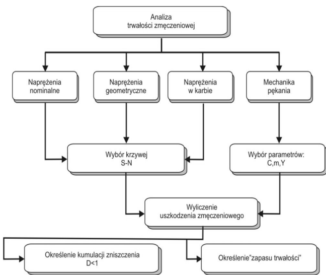
Rys. 1. Metodologia określania właściwości zmęczeniowych elementów konstrukcji zawierającej połączenia spawane [1]
