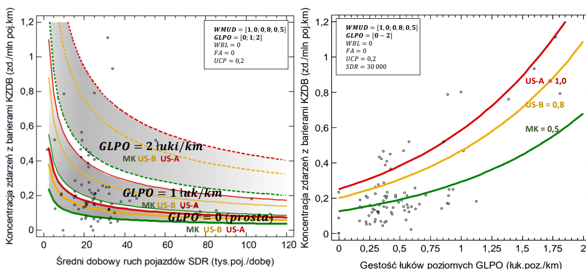
Rys. 9.13 Wpływ na koncentrację zdarzeń z barierami: a) natężenia ruchu (SDR) i gęstości łuków poziomych (GLPO) b) gęstości łuków poziomych (GLPO), względem współczynnika wykrywalności zdarzeń (WZA) modelu DS-2J-D3(1)
