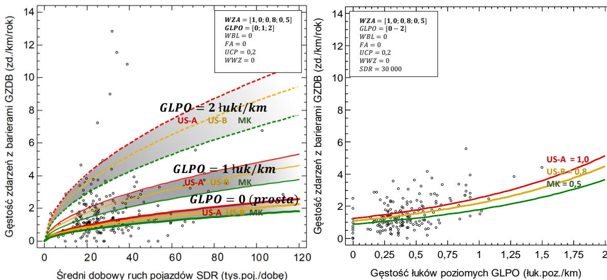
Rys. 9.7 Wpływ na gęstość zdarzeń z barierami: a) natężenia ruchu (SDR) i gęstości łuków poziomych (GLPO) b) gęstości łuków poziomych (GLPO), względem współczynnika wykrywalności zdarzeń (WZA) modelu DO-2J-C2(1)
