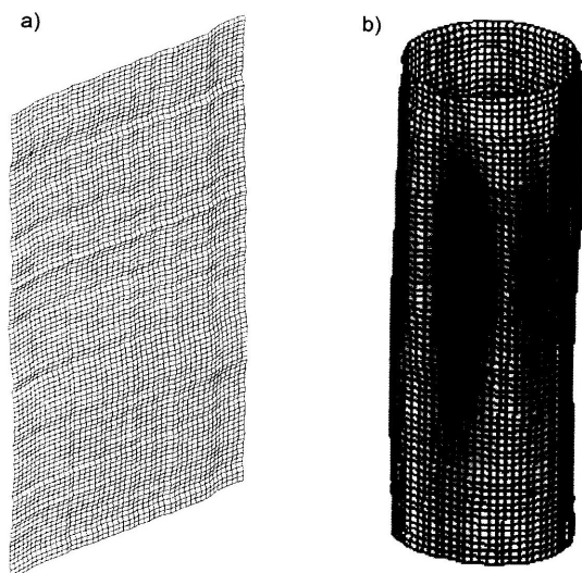
Rys. 4. Alumirowy silos: a) wygenerowane niejednorodne pole imperfekcji płaszczka, b) deformacja płaszczka w stanie granicznym
