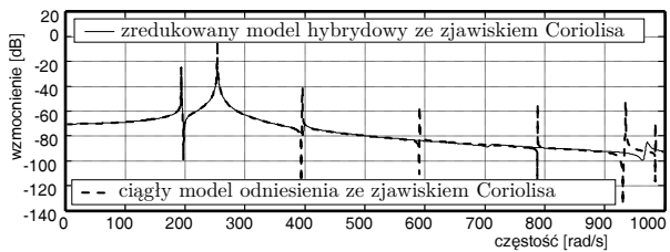
Rys. 9. Porównanie modelu hybrydowego struny z efektem Coriolisa z modelem referencyjnym (pochodna funkcji własnej mnożona przez siłę tarcia)
