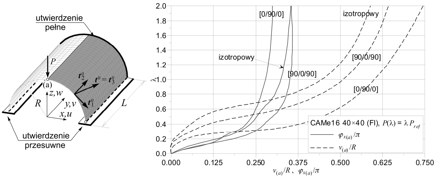
Rys.1 Cylindryczna powłoka obciążona siłą skupioną.
